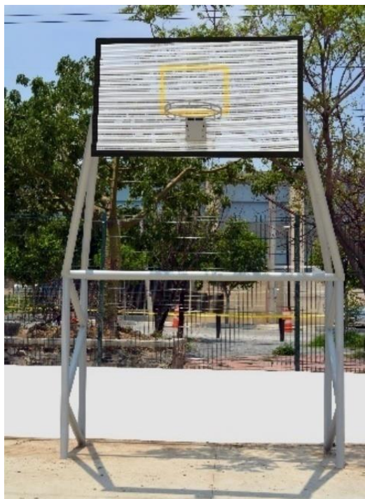
PORTERIA MULTIFUNCIONAL MODELO MM-MOSUL MEDIDAS: 4mts * 2.10mst * 1.00mts
